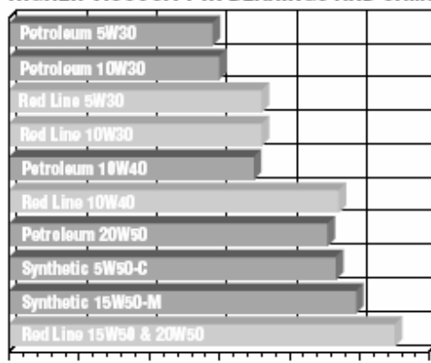
Figura 2: In presenza di alta velocità ed elevate temperature, Red Line Oil fornisce una viscosità significativamente superiore rispetto ai lubrificanti derivati dal petrolio. Red Line Oil fornisce una viscosità di grado più elevato rispetto a quella di un lubrificante derivato dal petrolio e di altri competitor sintetici.
