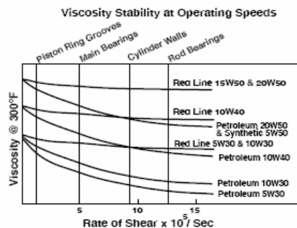
Figura 1: Red Line Oil 10W40 fornisce una protezione dei cuscinetti e delle bronzine più elevata rispetto a quella offerta dal lubrificante derivato dal petrolio 20W50. Notare come i lubrificanti derivati dal petrolio di alta qualità perdano una significativa parte della loro viscosità nei casi in cui vengano esposti a forze di elevata torsione sui cuscinetti e sulle pareti del cilindro.
